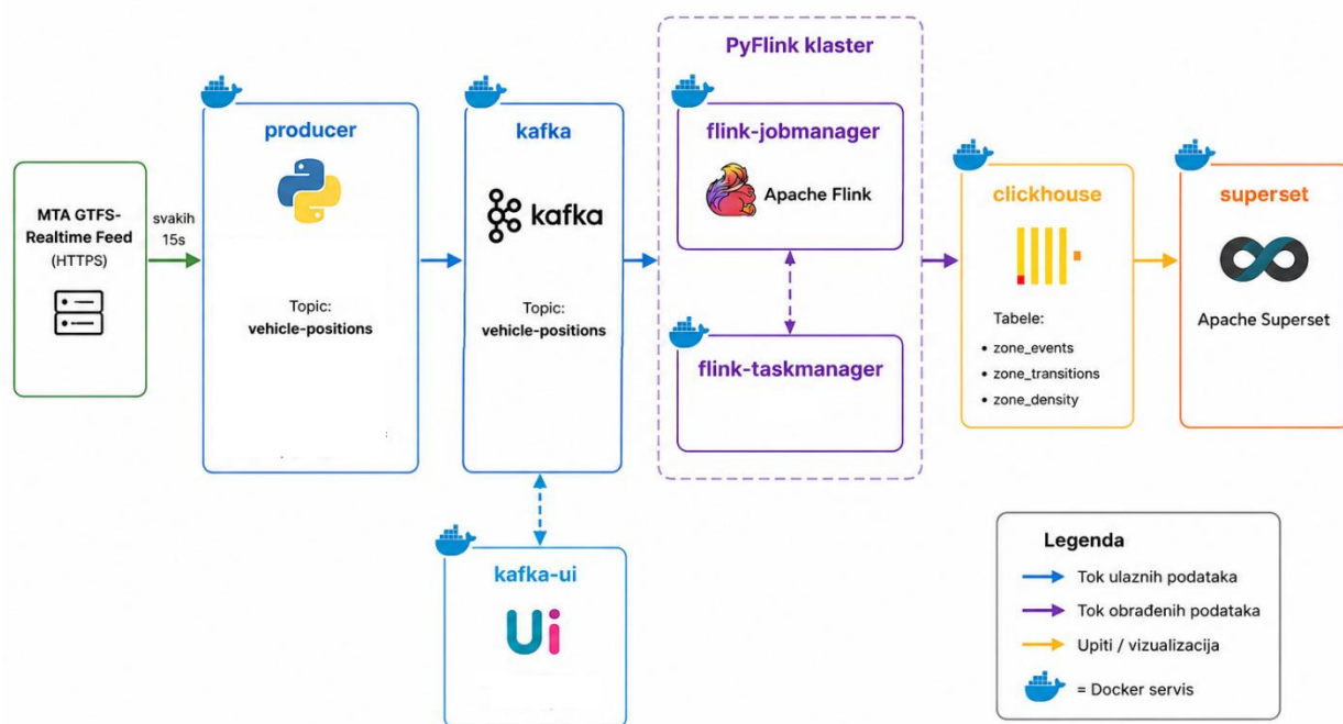
Slika 1. Dijagram arhitekture sistema
